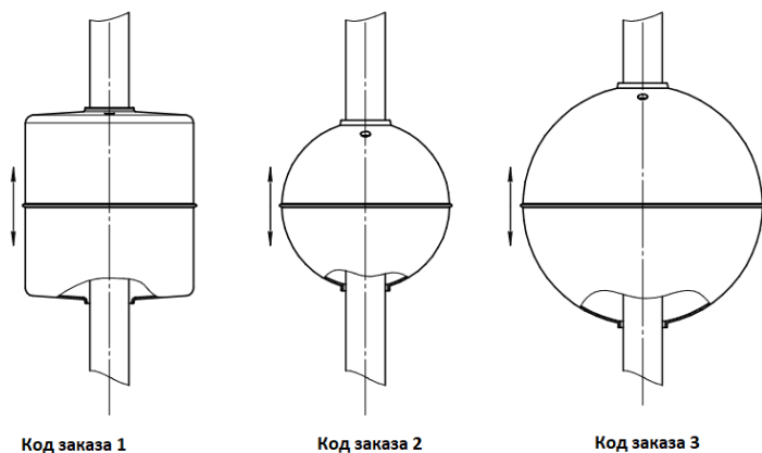
Рисунок 2.3 – Типы поплавков
