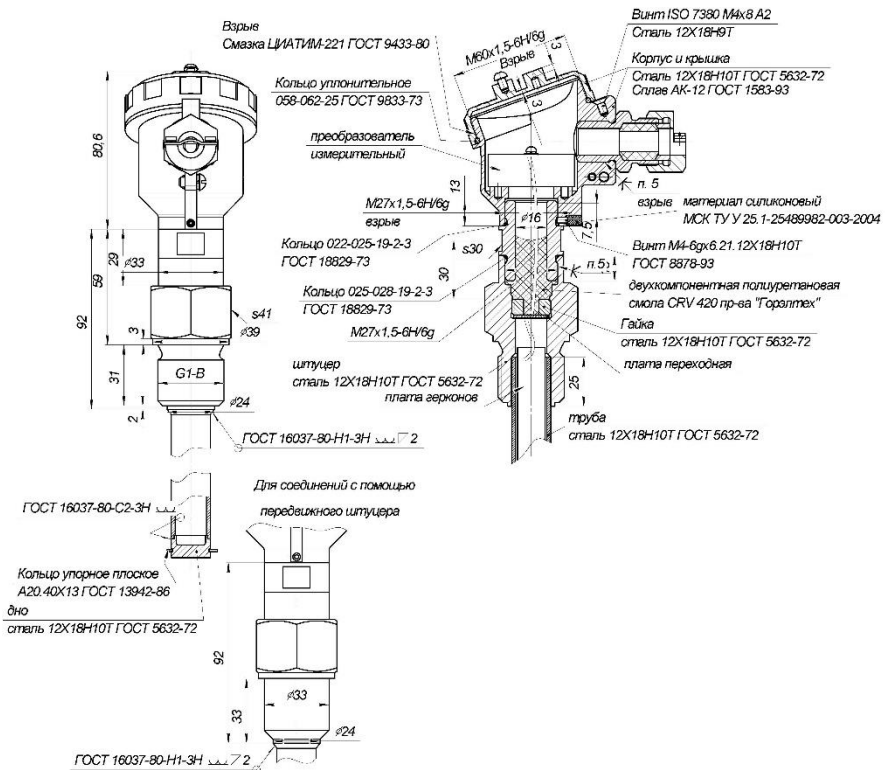
Рисунок А.5. - Чертеж обеспечения средств взрывозащиты УПП-11Exd/M2
